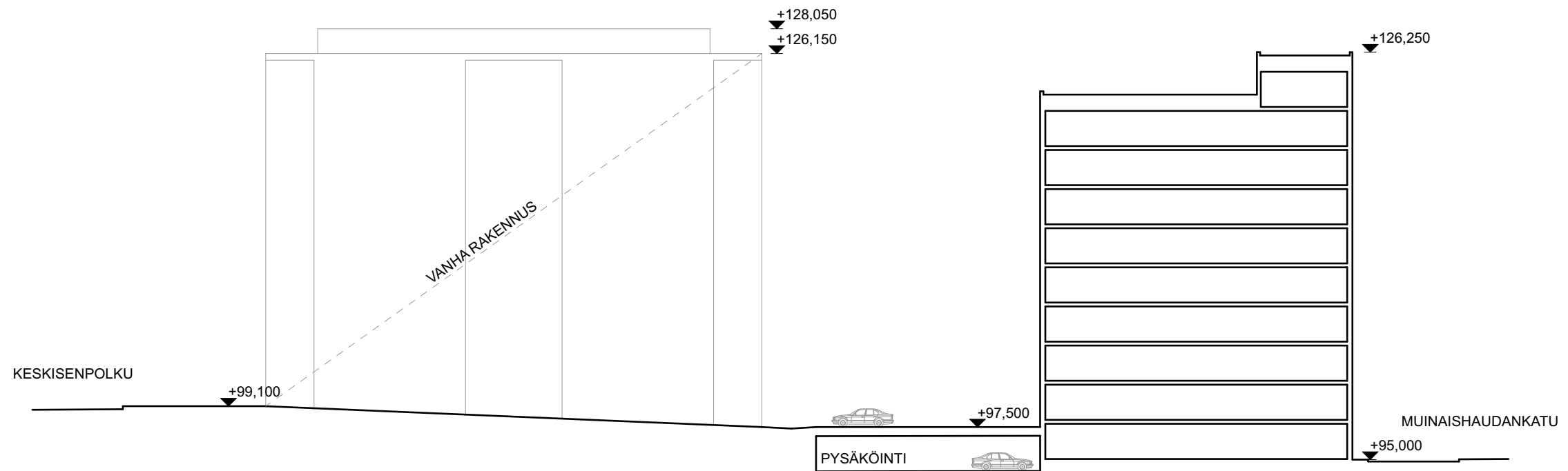
Leikkaus 1:400
