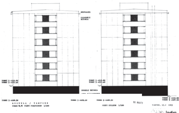
Kuva 65. Tornin 3 & 5 (6C & 8D) päätyjulkisivupiirroksiset pohjoiseen ja etelään vuodelta 1963. (Arkkitehtitoimisto Vahtera & Heino)
