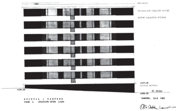
Kuva 64. Tornin 1 (2A) julkisivupiirros itään vuodelta 1963. (Arkkitehtitoimisto Vahtera & Heino)
