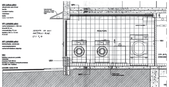
Kuva 26. Ote pesutuvan leikkauspiirrokselta vuodelta 2008. (Arkkitehdit A3 Oy)
