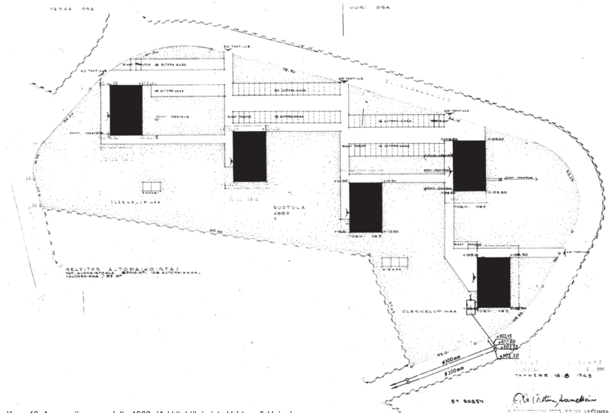
Kuva 19. Asemapiirros vuodelta 1963. (Arkkitehtitoimisto Vahtera & Heino)
