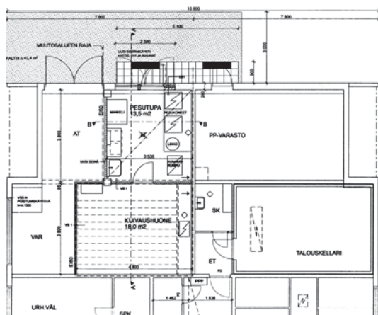
Kuva 24. Pohjapiirros pesutuvasta vuodelta 2008. (Arkkitehdit A3 Oy)
