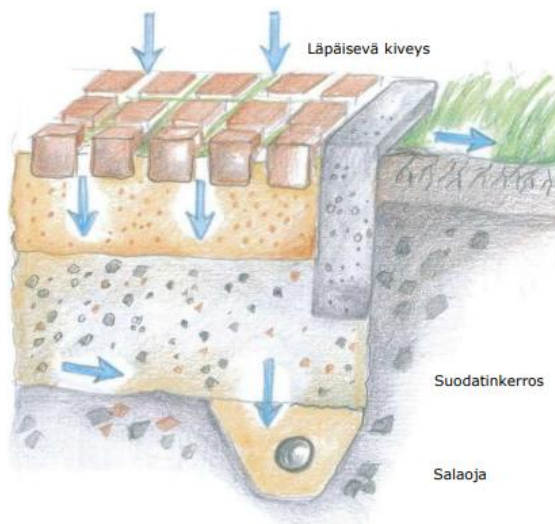
Kuva 5.2. Läpäisevä päällyste. Rakenteen päällä on läpäisevä kiveys, jonka alla on suodatinkerros. Rakente on salaojitettu.
