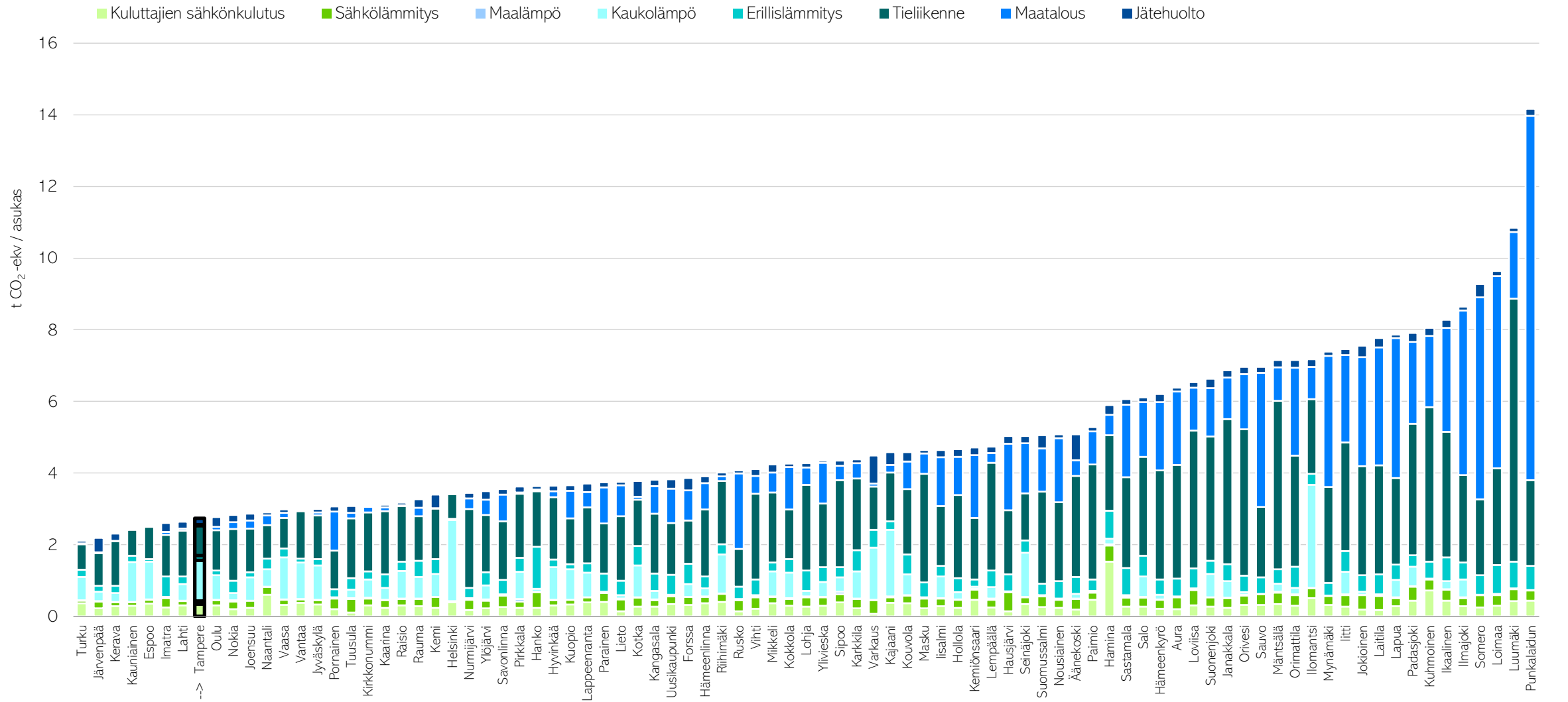
Kuva 18. Asukaskohtaiset päästöt (t CO 2 -ekv/asukas) kaikissa CO 2 -raportin kunnissa vuonna 2022 ilman teollisuutta. (CO 2 -raportti, 2024).
