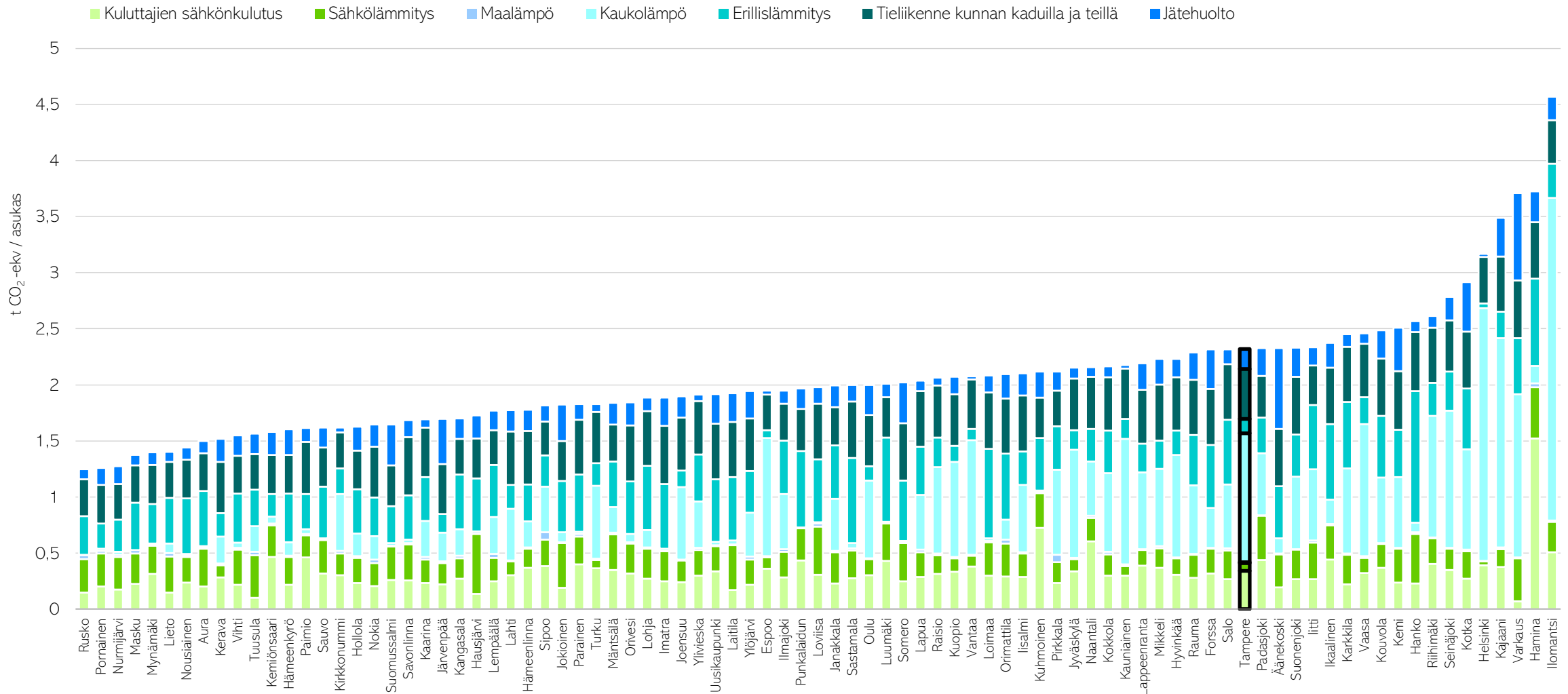
Kuva 19. Asukaskohtaiset päästöt (t CO 2 -ekv/asukas) kaikissa CO2-raportin kunnissa vuonna 2022 ilman teollisuutta, maataloutta ja läpiajoliikennettä. (CO 2 -raportti, 2024).
