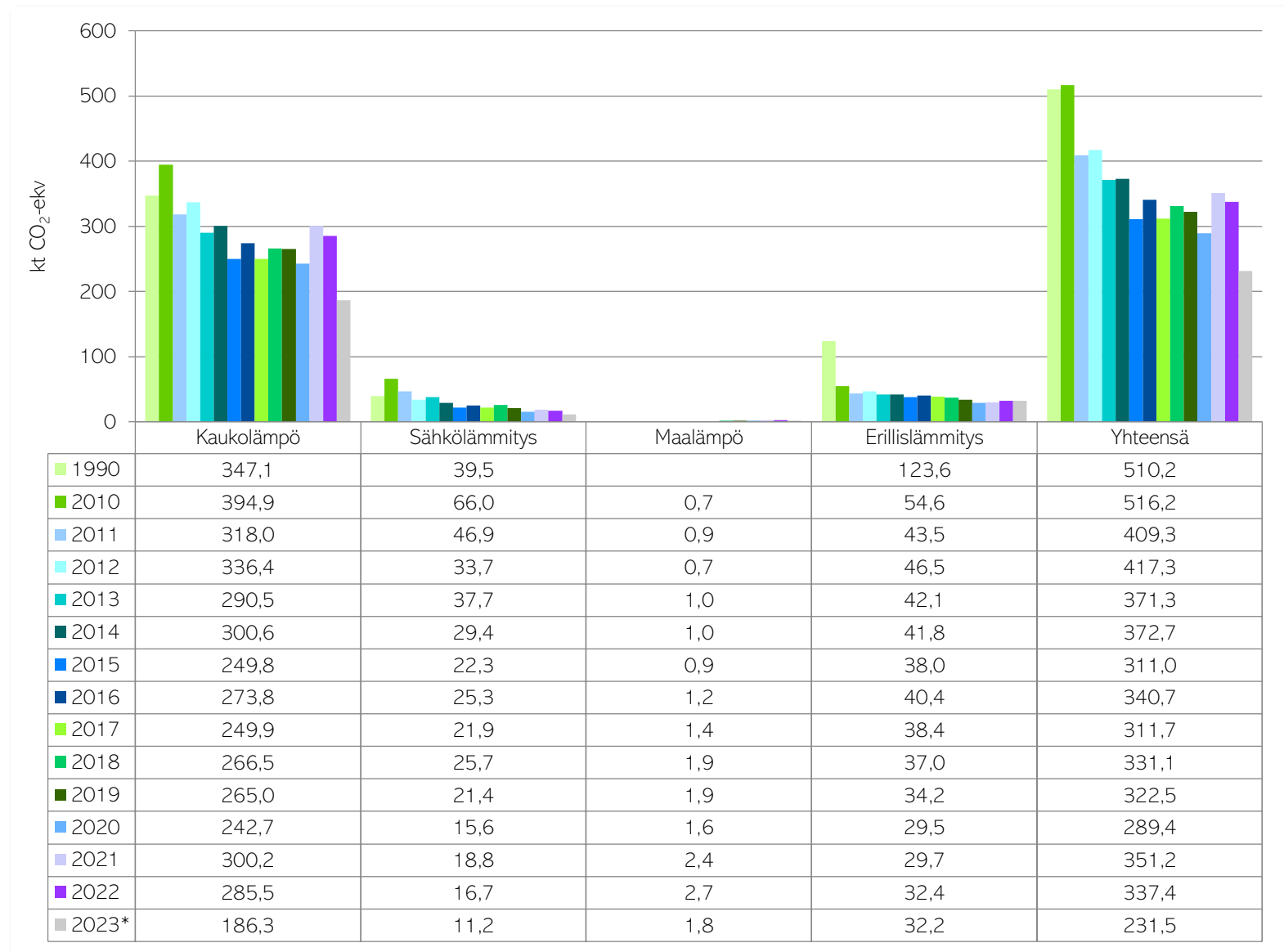
Kuva 8. Rakennusten lämmityksen päästöjen kehitys Tampereella vuonna 1990 ja vuosina 2010–2023. Vuoden 2023 tieto on ennakkotieto. (CO 2 -raportti, 2024).
