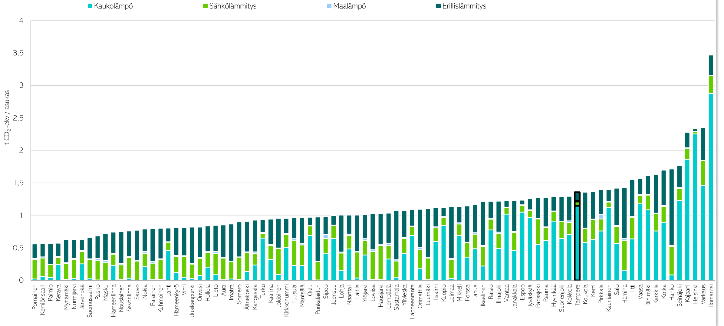
Kuva 20. Asukaskohtaiset päästöt (t CO 2 -ekv/asukas) lämmityksestä kaikissa CO 2 -raportin kunnissa vuonna 2022. (CO 2 -raportti, 2024).
