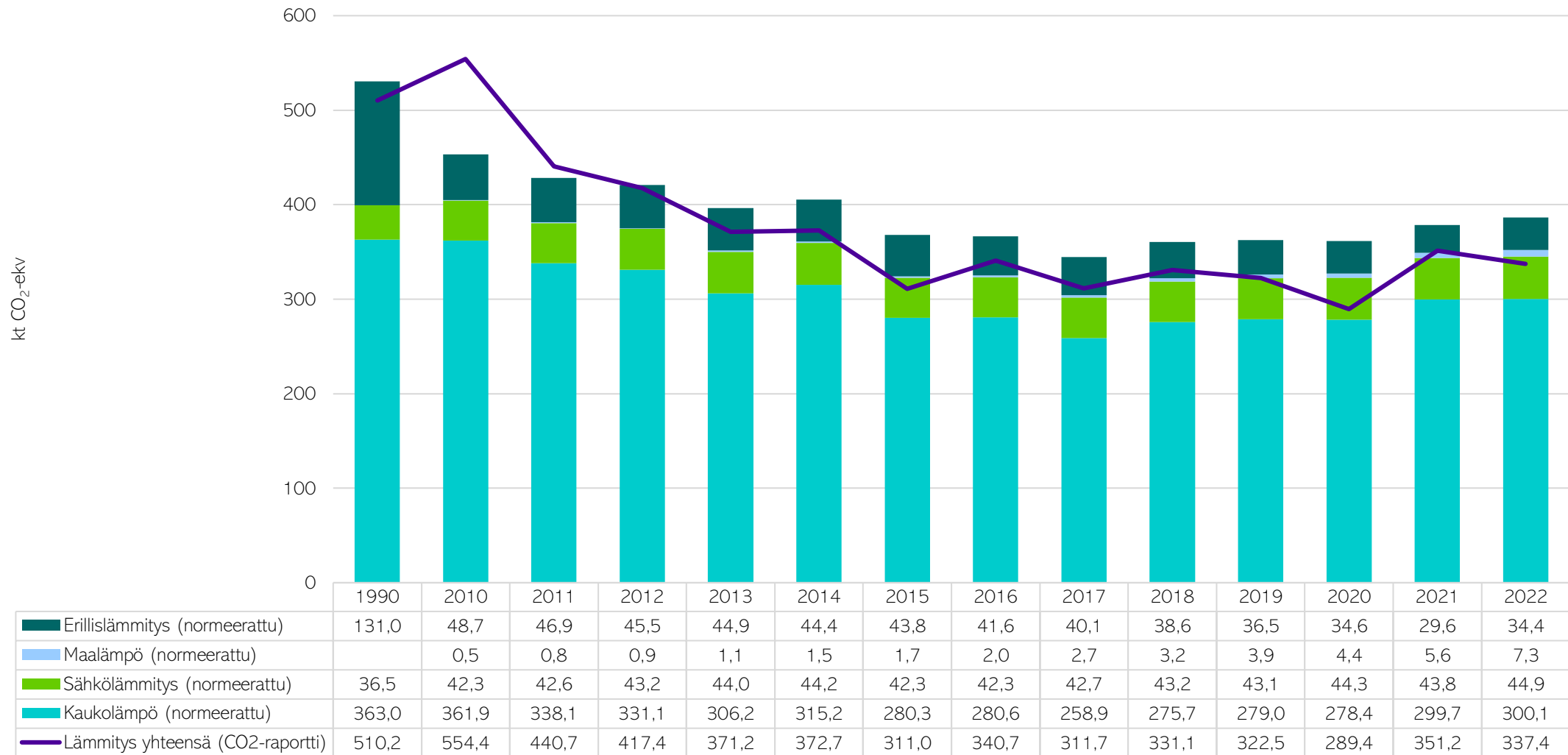
Kuva 9. Lämmityksen päästöt Tampereella vuonna 1990 ja vuosina 2010–2022 korjattuna vastaamaan ilmastollista vertailukautta 1981–2010 ja käyttäen sähkölämmitykselle ja maalämmölle keskimääräistä päästökerrointa. Normeeraamattomat CO2-raportin menetelmällä lasketut lämmityksen päästöt yhteensä on esitetty viivalla. (CO2-raportti, 2024).
