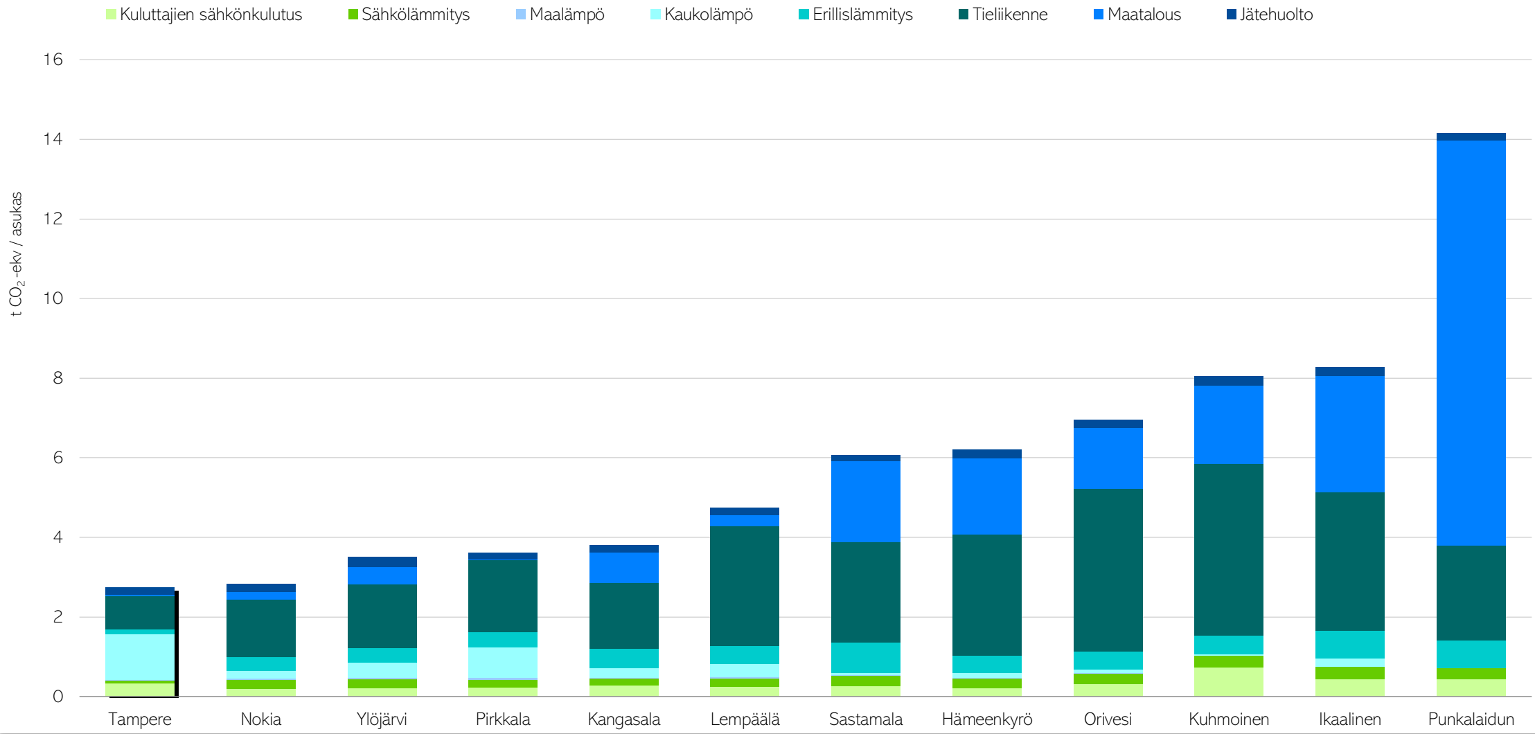
Kuva 14. CO2-raportissa mukana olevien Pirkanmaan kuntien asukaskohtaiset päästöt (t CO 2 -ekv/asukas) vuonna 2022 ilman teollisuutta. (CO 2 -raportti, 2024).
