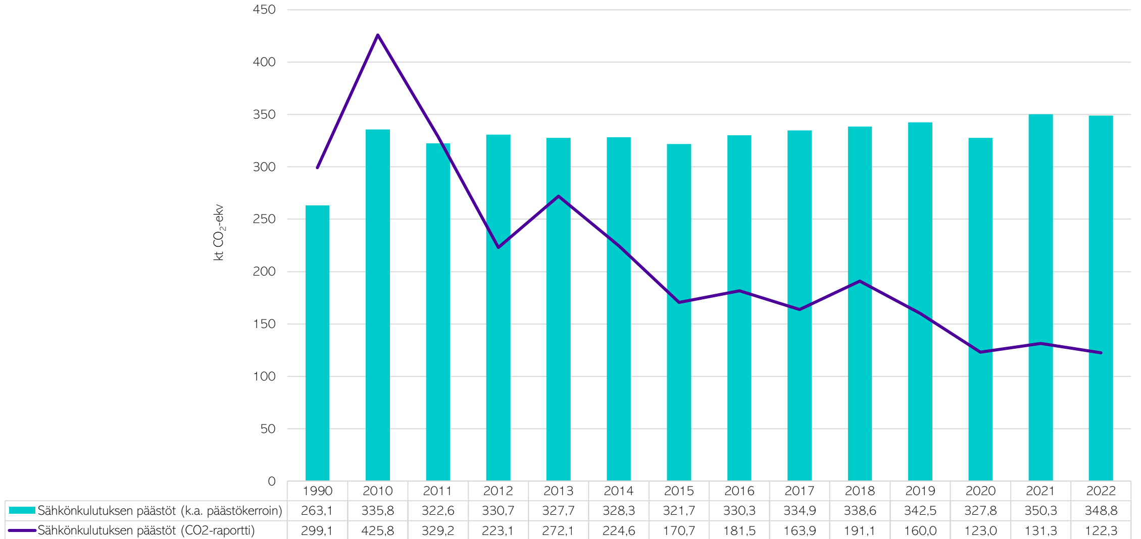
Kuva 7. Tampereen sähkönkulutuksen päästöt vuonna 1990 ja vuosina 2010–2022 (sisältäen kuluttajien ja teollisuuden sähkönkulutuksen, sähkölämmityksen ja maalämpöpumppujen sähkökäytön) laskettuna CO2-raportin menetelmällä (viiva) ja keskimääräistä päästökerrointa käyttäen (pylväät). (CO2-raportti, 2024).
