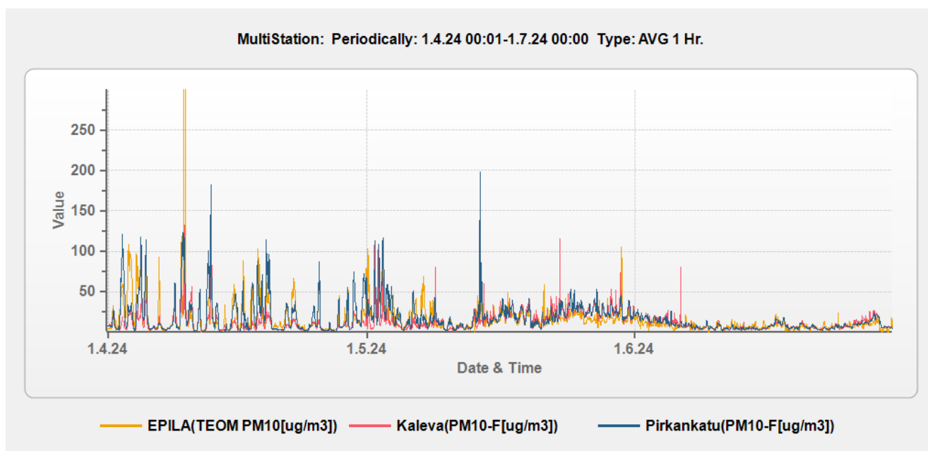
Kuva 2.3 Hengitettävien hiukkasten pitoisuuden tuntikeskiarvot Epilässä, Kalevassa ja Pirkankadulla mittausjakson aikana. (Suurin tuntikeskiarvo maaliskuussa Epilässä 530 \mu\text{g}/\text{m}^3 ).
