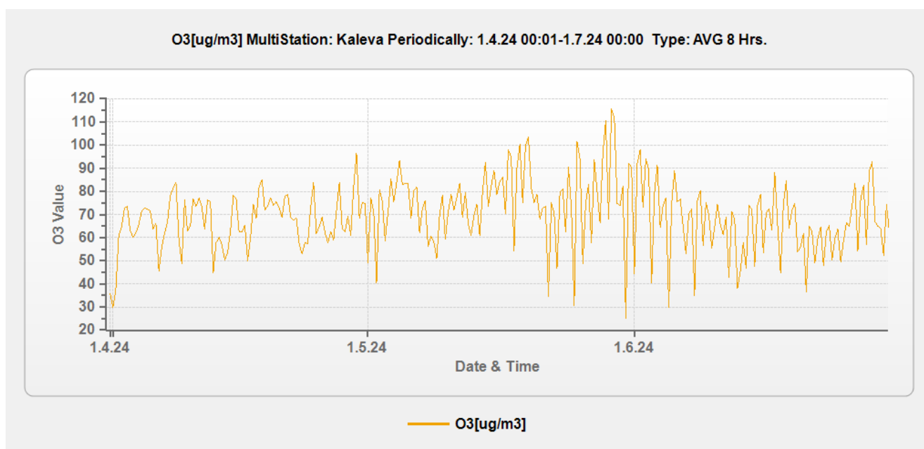
Kuva 6.1 Otsonipitoisuuden (ei-liukuvat) 8h-keskiarvot Kalevan mittausasemalla.
