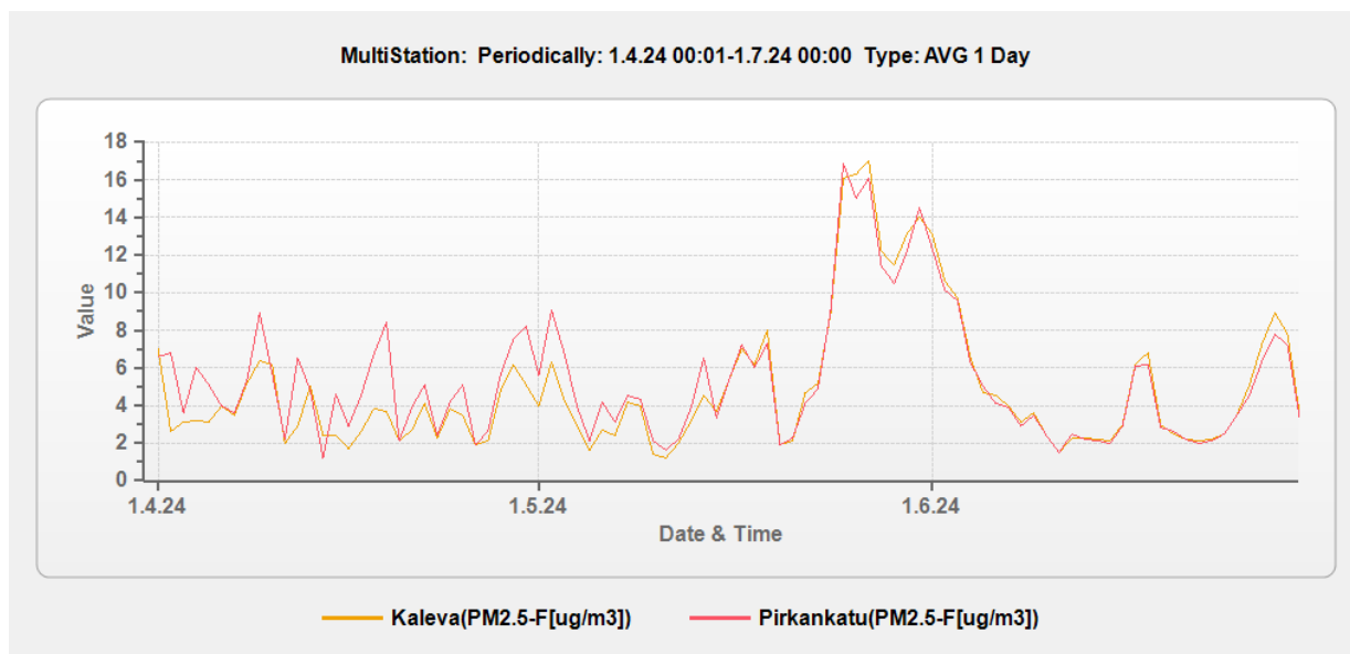
Kuva 3.3 Pienhiukkasten pitoisuuden vuorokausikeskiarvot mittausjakson aikana Kalevassa ja Pirkankadulla (Fidas).
