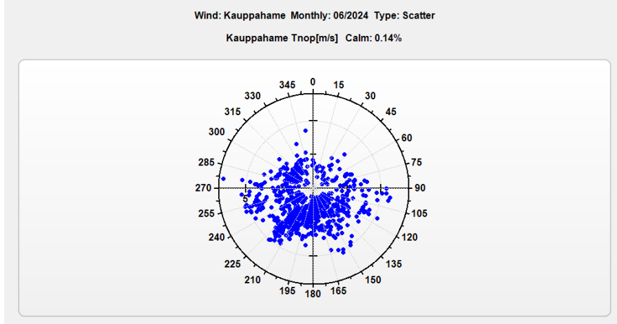
Kuva 7.2 Tuulen nopeus suunnittain 1h keskiarvoina Kauppa-Hämeen sääasemalta.
