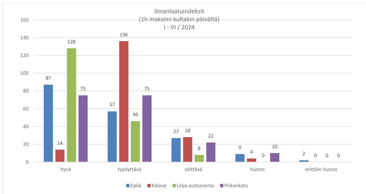
Kuva 8.1. Yhteenveto ilmanlaadusta Tampereen eri asemilla (kunkin päivän 1 tunnin indeksien maksimiarvon perusteella) kuluneen vuoden aikana. Kaupunkitausta-asemalla Kalevassa otsonipitoisuus (jota muilla asemilla ei mitata) vähentää varsinkin kesäkaudella Kalevassa hyväksi luokitettujen päivien lukumäärää.
