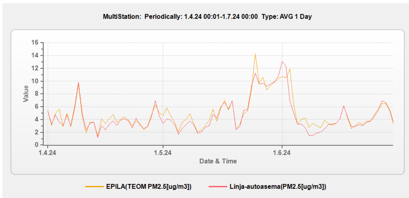
Kuva 3.1 Pienhiukkasten pitoisuuden vuorokausikeskiarvot mittausjakson aikana Epilässä ja Linja-autoasemalla (Teom).
