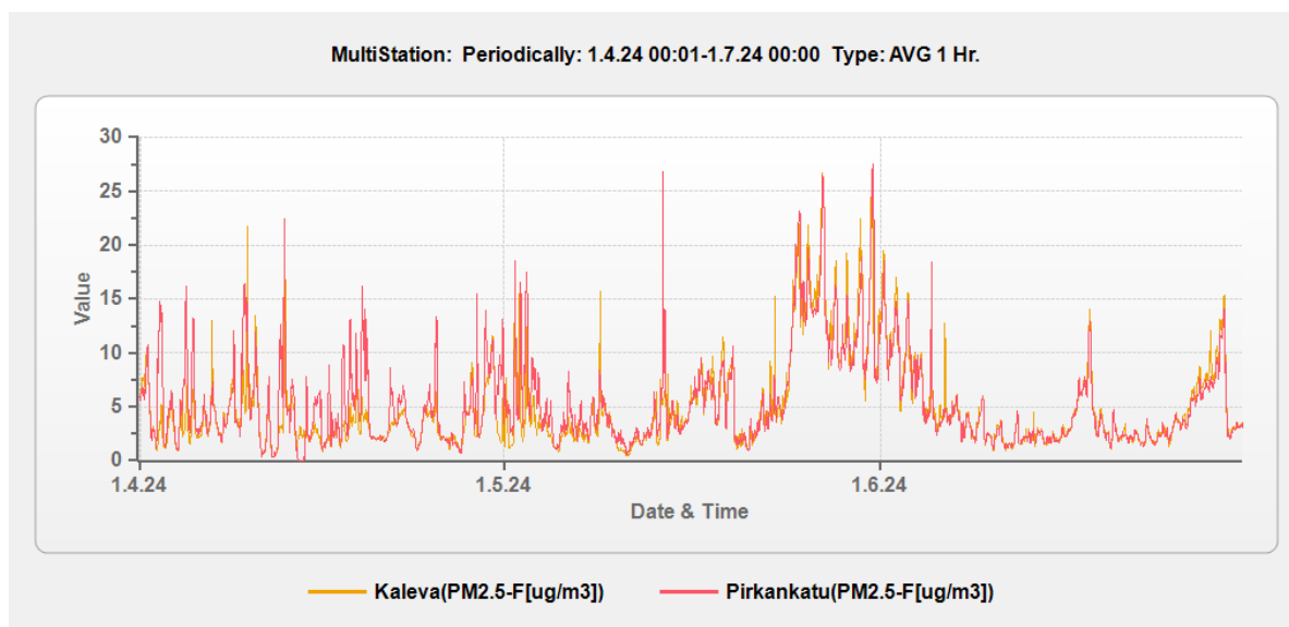
Kuva 3.4 Pienhiukkasten pitoisuuden tuntikeskiarvot mittausjakson aikana Kalevassa ja Pirkankadulla (Fidas).
