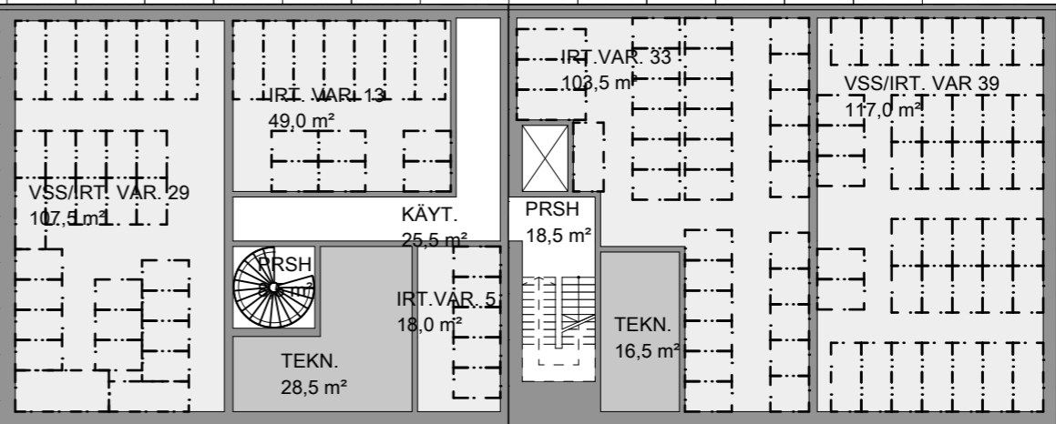
PELTOTALO 1
