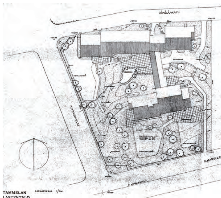
Asemapiirros vuodelta 1951/ Tapani Nironen.
