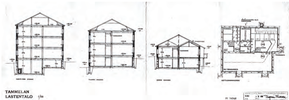
Kellarikerros v. 1951.
