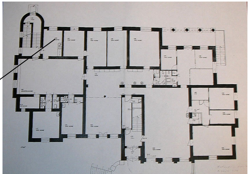
Pohjapiirros 1. krs
