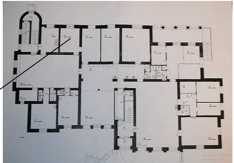
Pohjapiirros 1. krs
