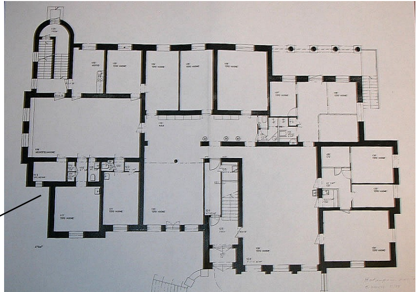
Pohjapiirros 1. krs
