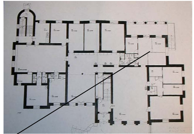
Pohjapiirros 1.krs
