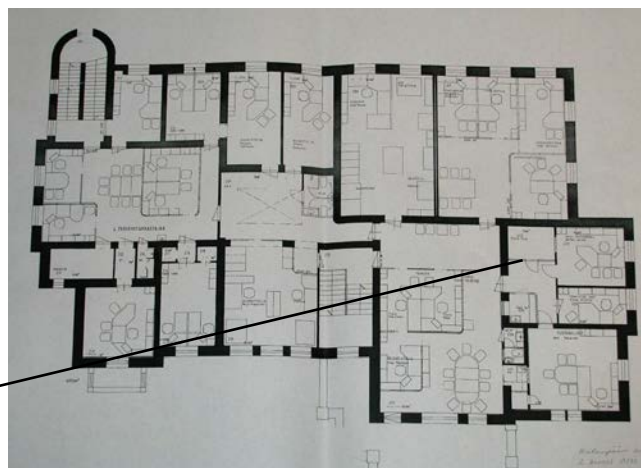
Pohjapiirros 2.kerros
