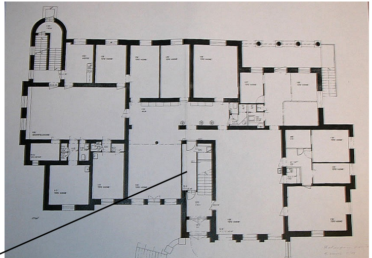
Pohjapiirros 1. krs
