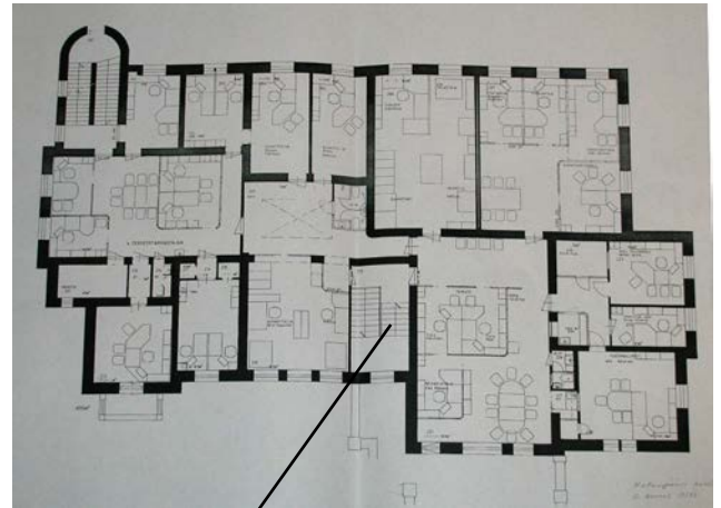
Pohjapiirros 2.kerros
