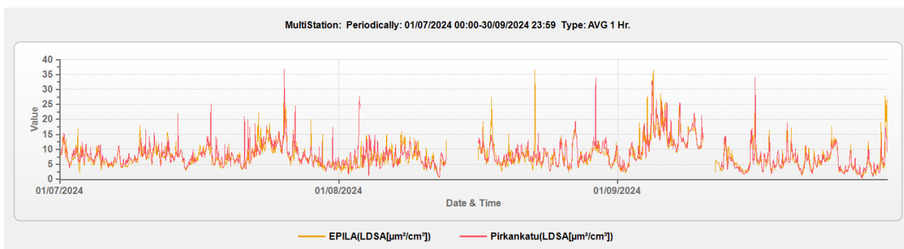
Kuva 4.3 Hiukkasten keuhkodepositiivan pinta-alan (LDSA) tuntikeskiarvoja ( \mu\text{m}^2/\text{cm}^3 ) Epilän ja Pirkankadun mittausasemilta.
