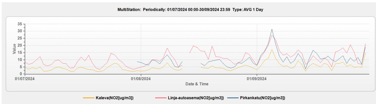
Kuva 5.1a Typpidioksidin pitoisuuden vuorokausikeskiarvot eri mittausasemilla mittausjakson aikana.
