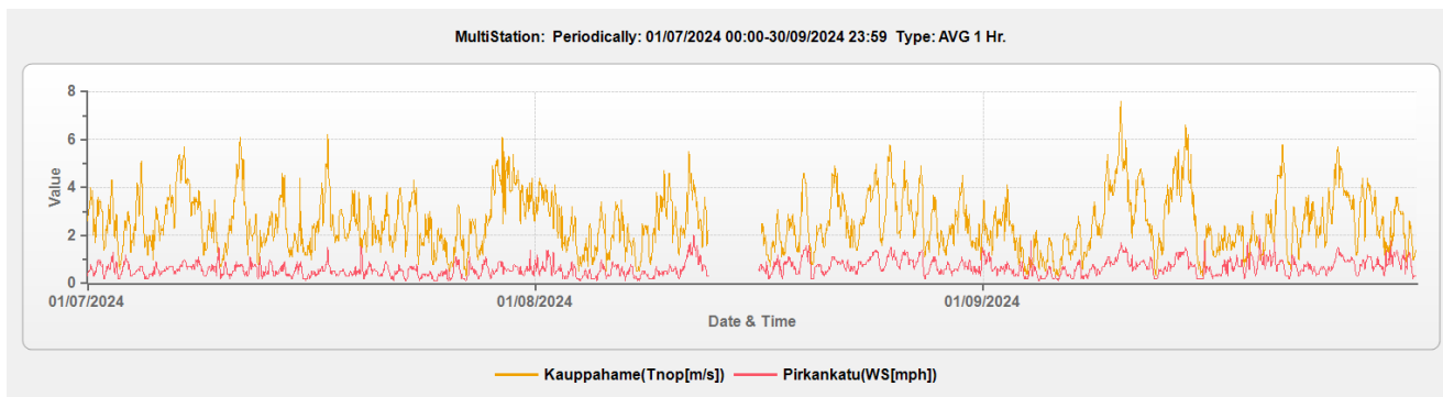
Kuva 7.3 Tuulen nopeuden 1h keskiarvot Kauppa-Hämeen ja Pirkankadun sääasemilta.
