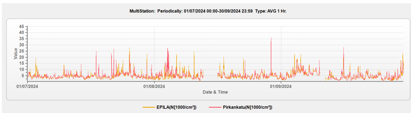
Kuva 4.5 Hiukkasten lukumääräpitoisuuden tuntikeskiarvoja ( 1000 \text{ kpl/cm}^3 ) Epilän ja Pirkankadun mittausasemilta.
