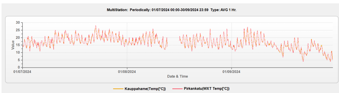
Kuva 7.3 Lämpötilan tuntikeskiarvot Kauppa-Hämeen ja Pirkankadun sääasemilta.
