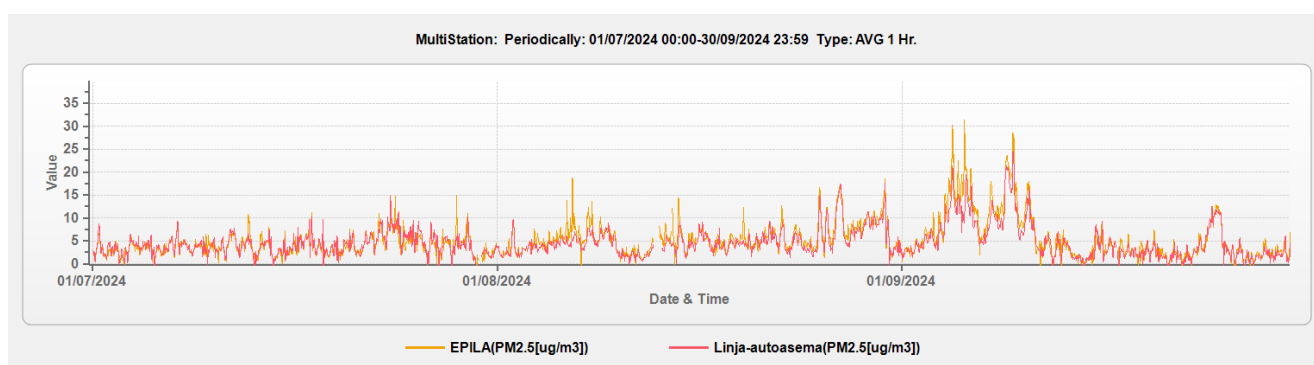
Kuva 3.2 Pienhiukkasten pitoisuuden tuntikeskiarvot mittausjakson aikana Epilässä ja Linja-autoasemalla (Teom).
