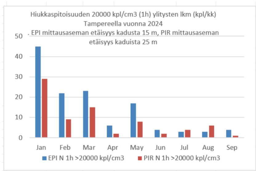
Kuva 4.6 Hiukkaspitoisuuden 20000 \text{ kpl/cm}^3 (1h) ylitysten lukumäärät Epilän ja Pirkankadun mittausasemilla vuonna 2024. Esim. tammikuussa Epilässä (WHO:n 2021 kannanoton mukaisesti) kyseisen, korkeaksi katsottavan (taulukko 4.1) pitoisuustason ylityksiä oli 45 kpl.
