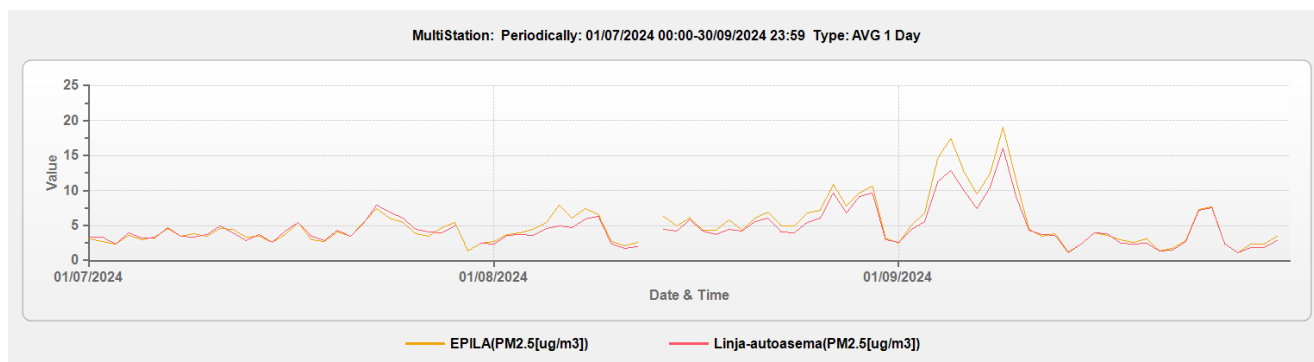
Kuva 3.1 Pienhiukkasten pitoisuuden vuorokausikeskiarvot mittausjakson aikana Epilässä ja Linja-autoasemalla (Teom).
