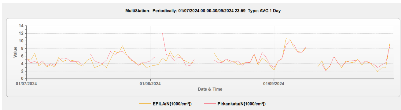
Kuva 4.4 Hiukkasten lukumääräpitoisuuden vuorokausikeskiarvoja ( 1000 \text{ kpl/cm}^3 ) Epilän ja Pirkankadun mittausasemilta.
