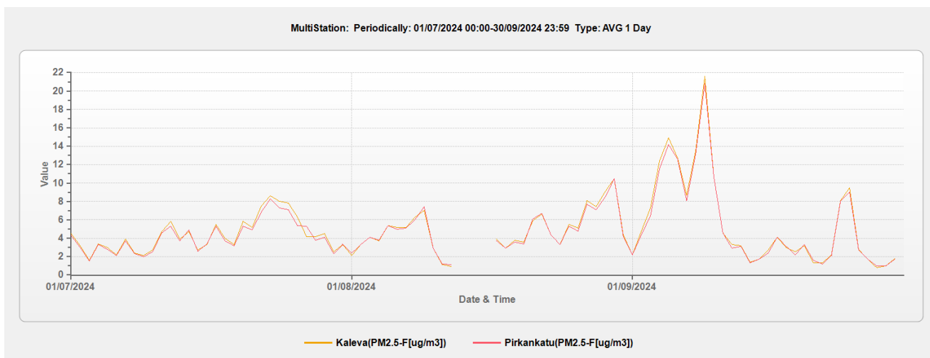
Kuva 3.3 Pienhiukkasten pitoisuuden vuorokausikeskiarvot mittausjakson aikana Kalevassa ja Pirkankadulla (Fidas).
