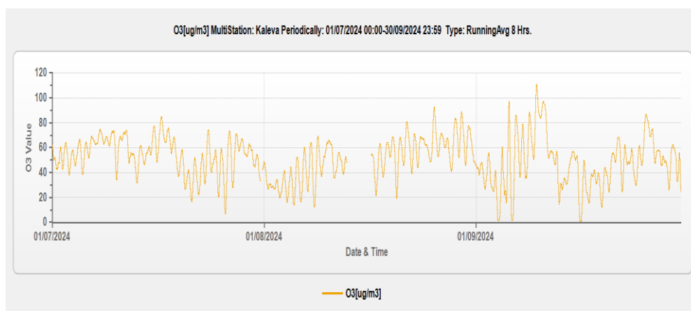
Kuva 6.1 Otsonipitoisuuden (liukuvat) 8h-keskiarvot Kalevan mittausasemalla.
