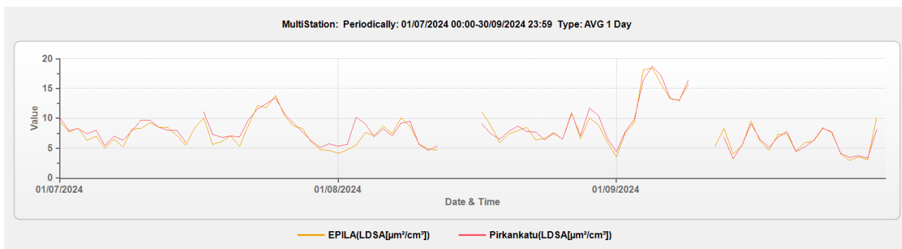
Kuva 4.2 Hiukkasten keuhkodepositiivan pinta-alan (LDSA) vuorokausikeskiarvoja ( \mu\text{m}^2/\text{cm}^3 ) Epilän ja Pirkankadun mittausasemilta.
