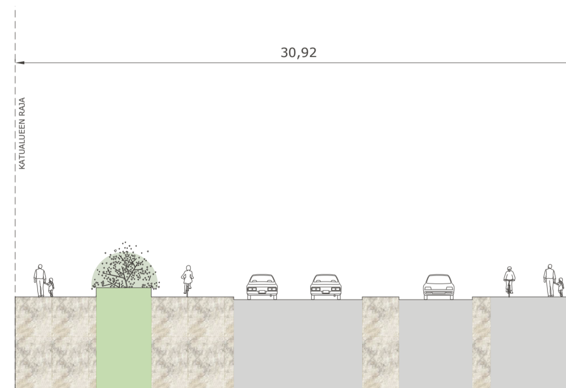
Leikkaus D-D
