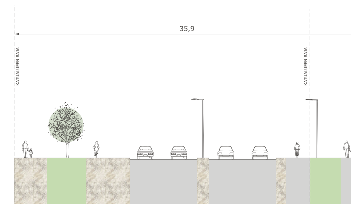
Leikkaus E-E
