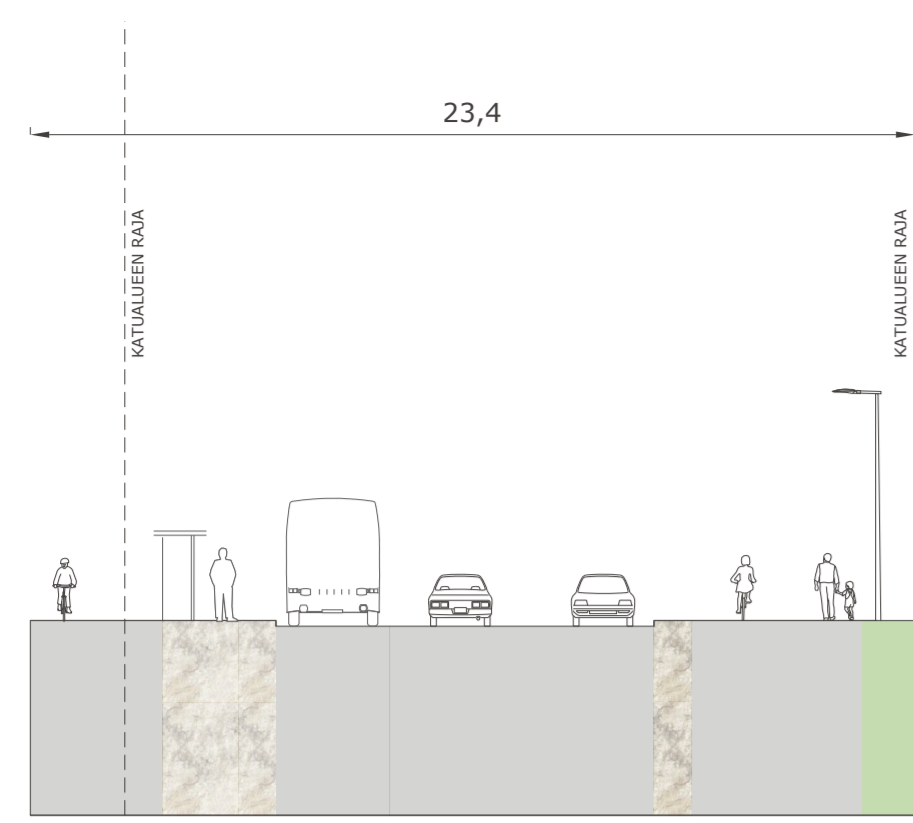
Leikkaus A-A
