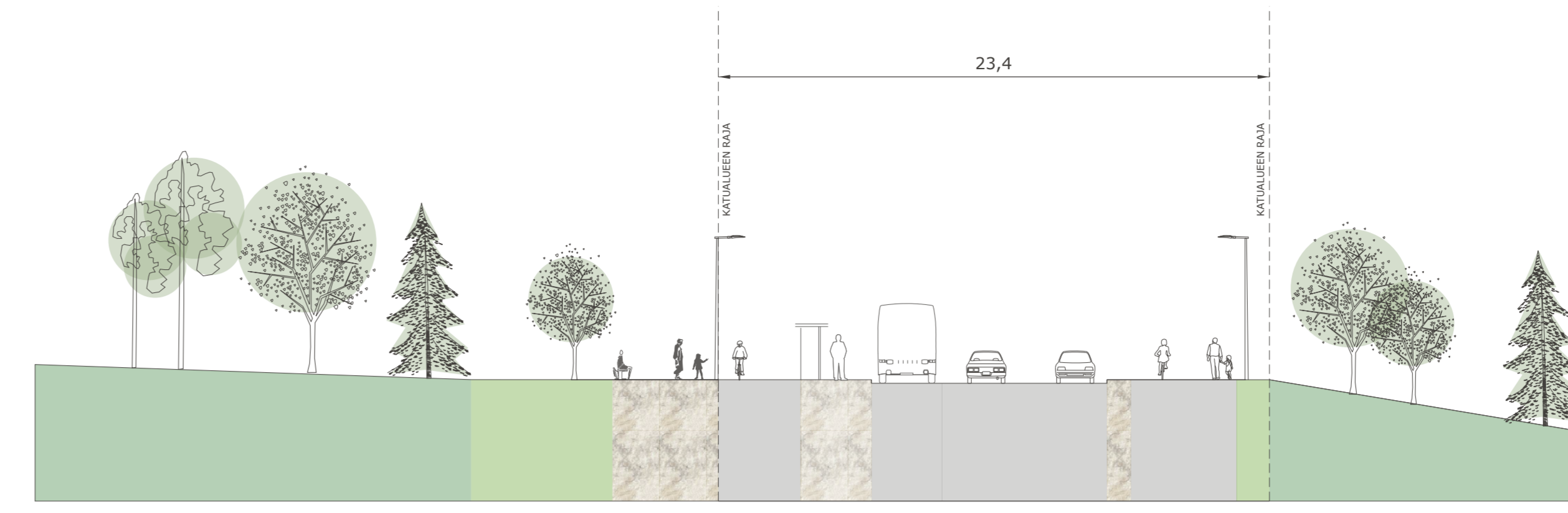
Leikkaus C-C
