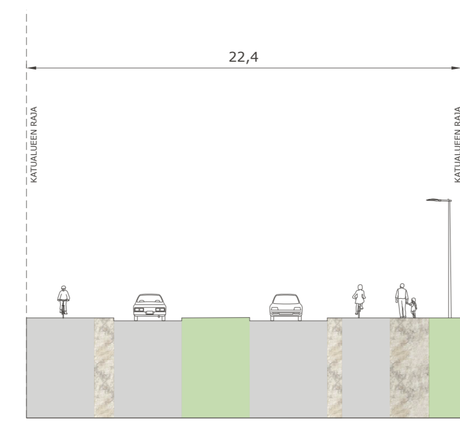
Leikkaus B-B
