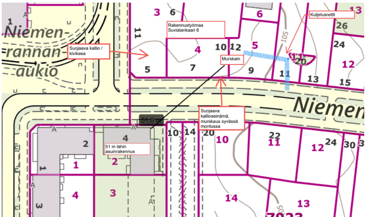
Kuva 1: Työmaan toimintojen sijoittuminen.
